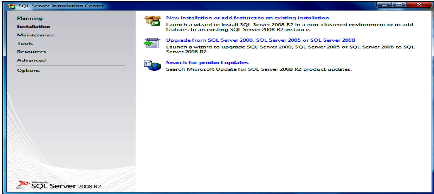
รูป หน้าจอหลักของโปรแกรมติดตั้ง Microsoft SQL Server 2008R2 Express
